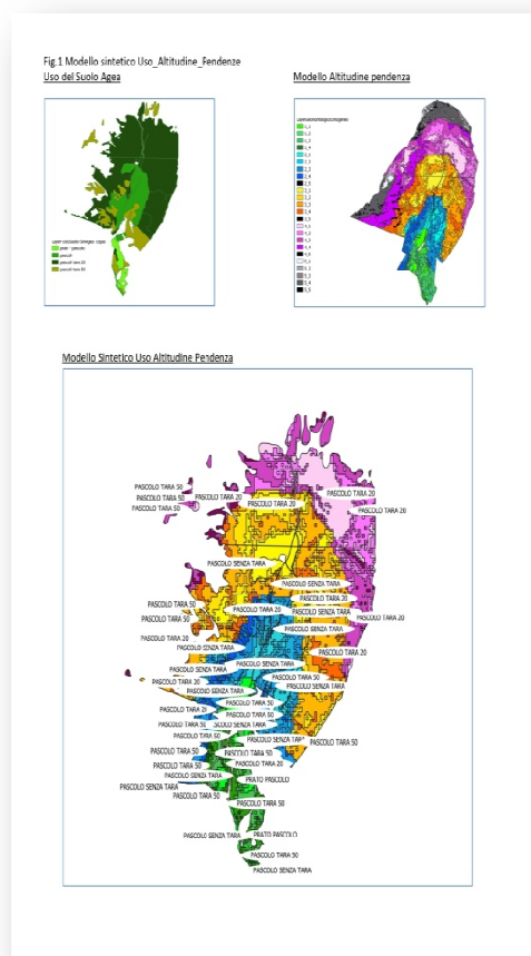
Fig. 1 Modèle synthétique Utilisation du sol_Altitude_Pente
