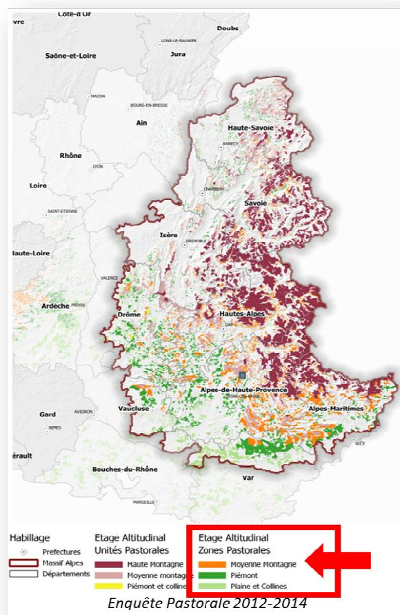
Figure 1 – Localisation des zones pastorales à l’échelle des Alpes françaises selon le recensement de l’Enquête Pastorale 2012-2014. Source: Enquête Pastorale 2012-2014.
