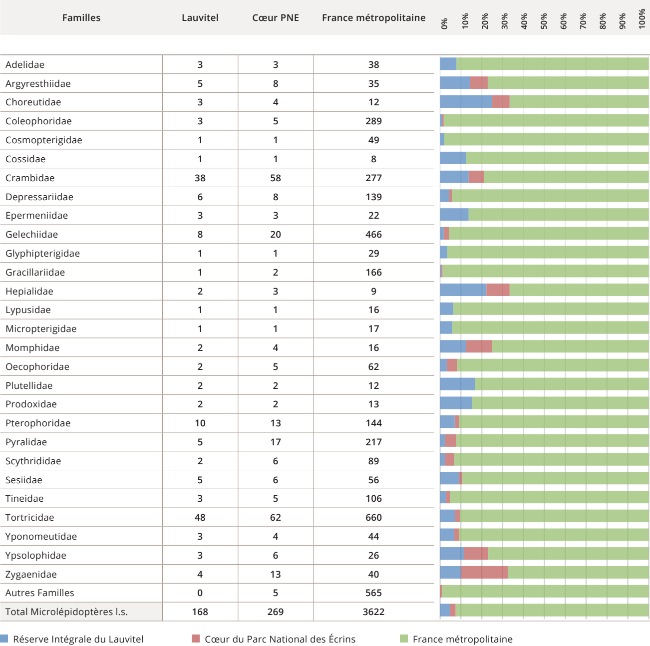
Figure 12. Bilan par famille du nombre d'espèces de Microlépidoptères l.s. citées sur la Réserve Intégrale du Lauvitel par rapport au Cœur du Parc National des Écrins et la France métropolitaine.
