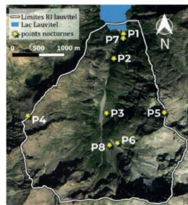
Fig. 4 : localisation des placettes d'inventaires nocturnes (emplacement du piège cloche). ►
