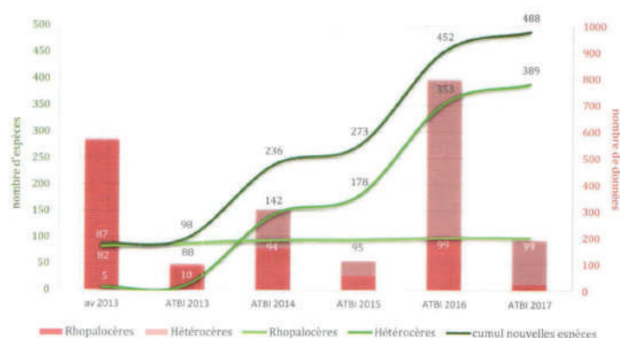
Fig. 10 : évolution annuelle des données récoltées.
