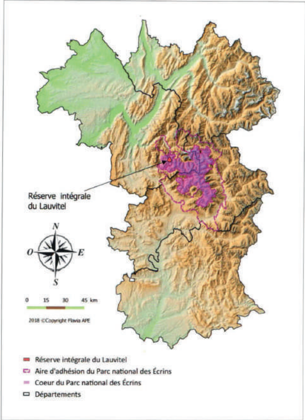
Fig. 1: la réserve intégrale du Lauvitel au sein du système alpin français.
